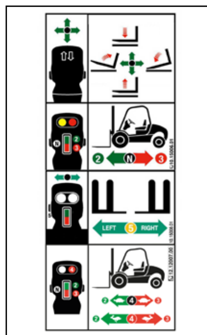
(fig. 5) MÁQUINA CON VELOCIDAD RÁPIDA MARCHA ATRÁS
